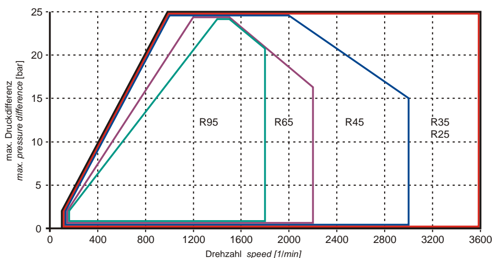
Abb. 4: Zulässige Druckdifferenz (Viskosität 33 mm 2 /s)
